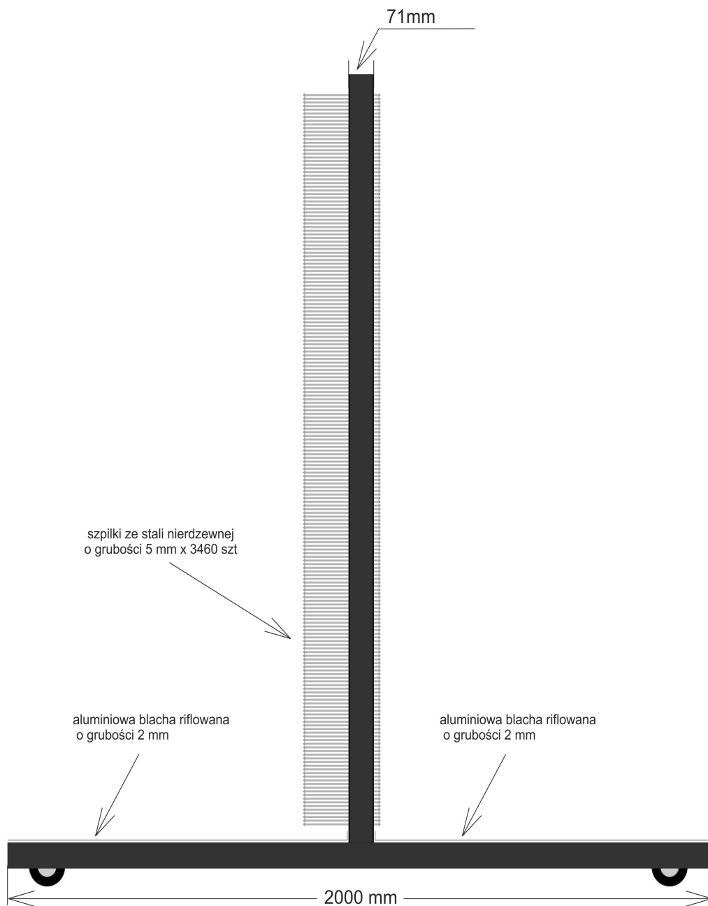
Rys. 1 Rzut z boku
